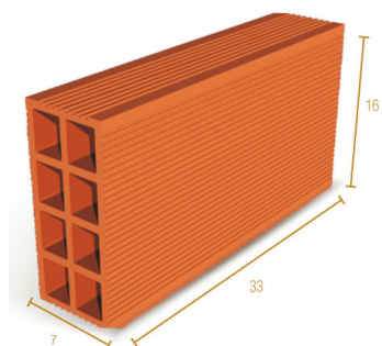
RASILLON DOBLE 33X16X7
