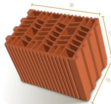
TERMOCERÁMICA 30X19X19
