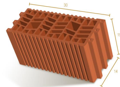
TERMOCERÁMICA 30X19X14
