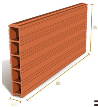
BARDO 80X25X3,5
