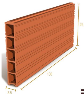
BARDO 100X25X3,5
